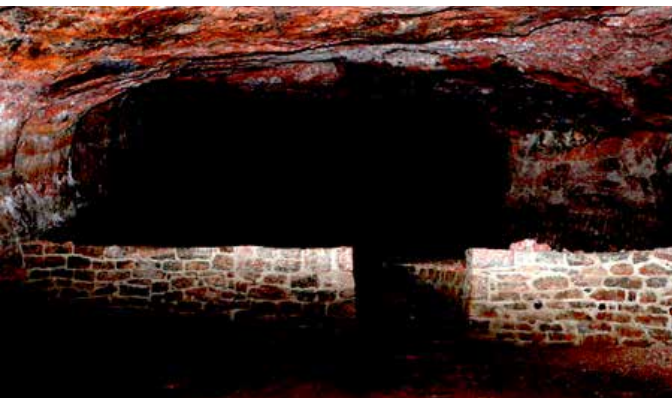
Abbaukammer im geschichteten Carnallitit in 620 m Tiefe unter der Feldflur östlich des ehemaligen Förderschachtes.
